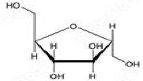
Beta-D-Fructose
