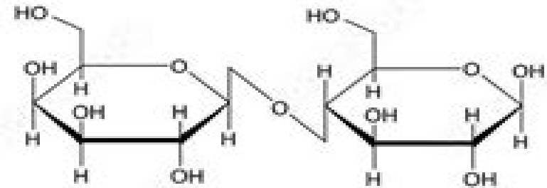
Lactose
