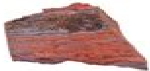
ferruginous quartzite (jaspillite)
