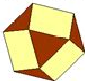
Kuboktaeder
