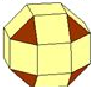
Rhombenkuboktaeder
