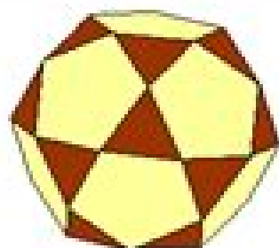
Ikosidodekaeder
