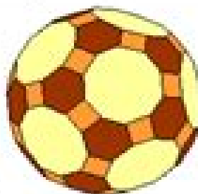
abgestumpftes Ikosidodekaeder
