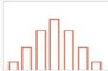
Binomial distribution
