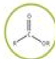
ESTER
