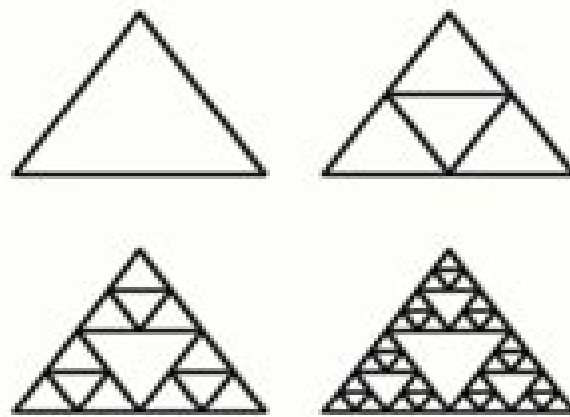
Sierpinski triangular
