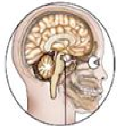
Craniopharyngiomas
