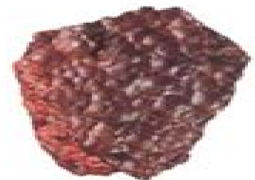
Hematite
