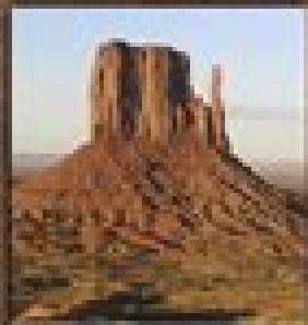
butte
