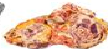
bauxite
