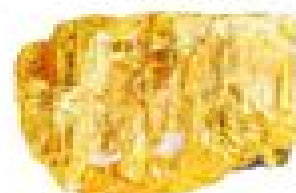
orpiment
