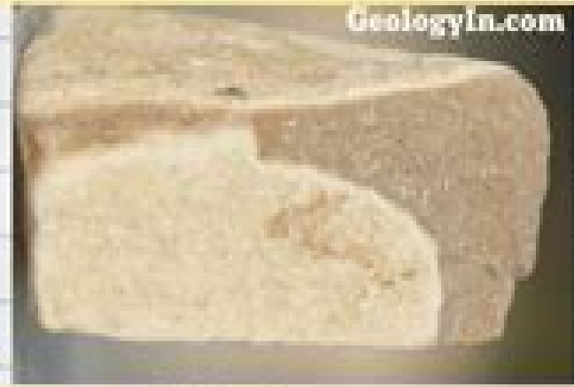
Mudstone
