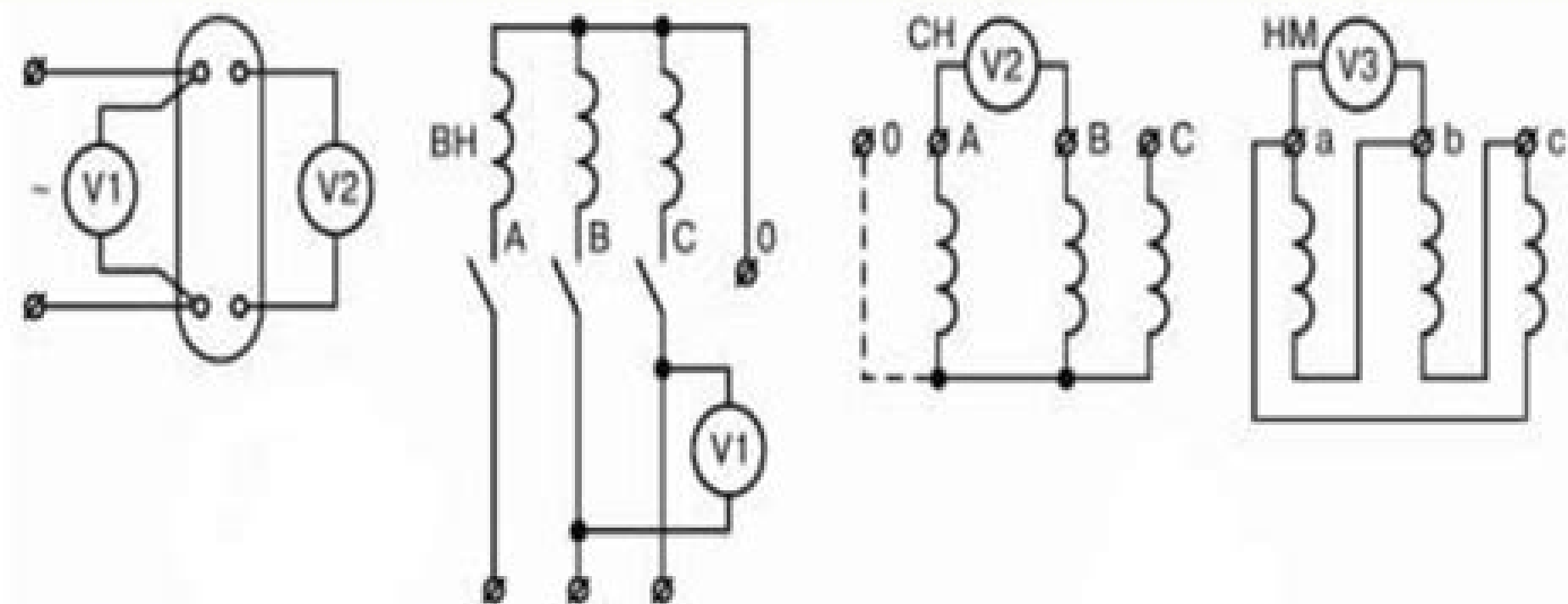
Рис. 1 - Метод двух вольтметров для определения коэффициентов трансформации: а – для двухобмоточных и б – трехобмоточных трансформаторов
