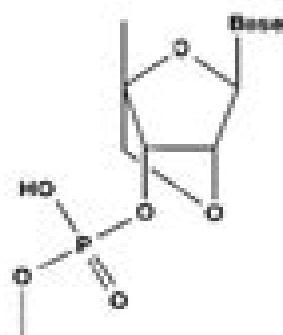
LNA 2',4'-BNA
