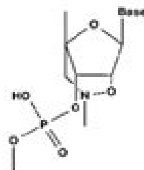
BNA HC
