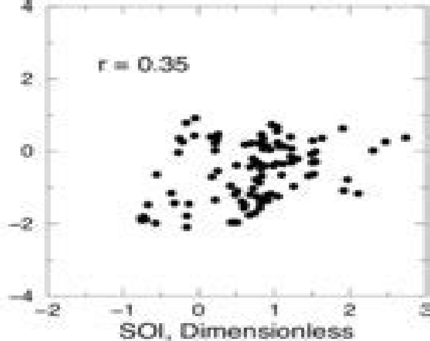
(d) 1960–84 SOI vs. RPC 5
