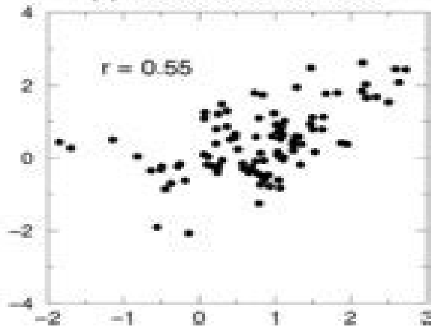
(d) 1960–84 SOI vs. RPC 5
