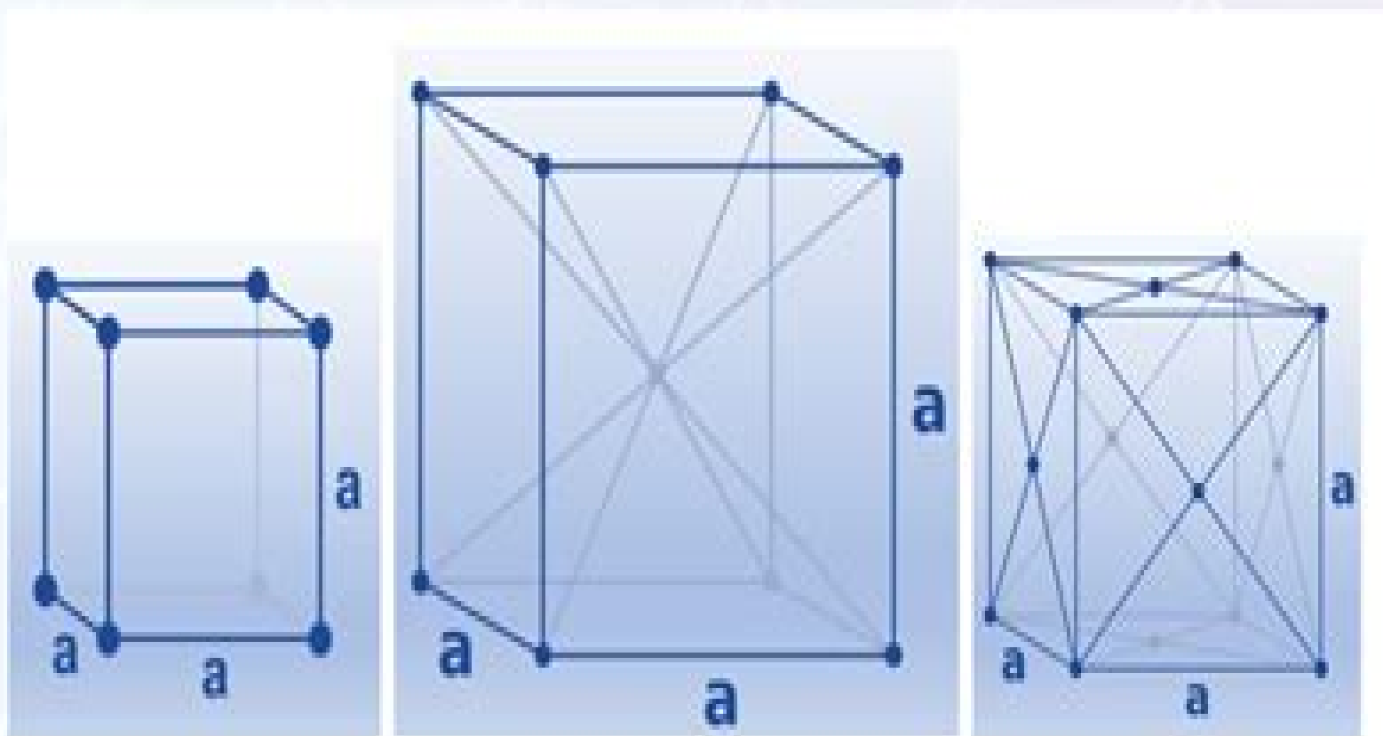
Simple Cubic
