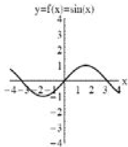
Sine Function
