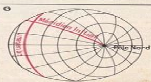
Fig. G. — Autre aspect du globe terrestre avec le réseau complet des méridiens et des parallèles, pour un observateur placé face au pôle Nord.
