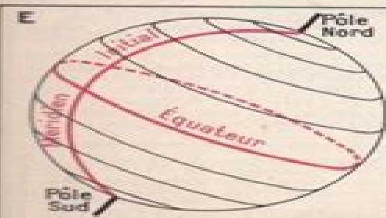
Fig. E. — Aspect de la terre, pour un observateur placé face à l'Équateur, si l'on avait tracé les parallèles sur le globe terrestre.
