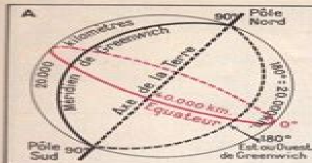
Fig. A. — On y voit l'axe de la terre, le méridien initial ou de Greenwich, point de départ des longitudes, et l'Équateur, point de départ des latitudes.
