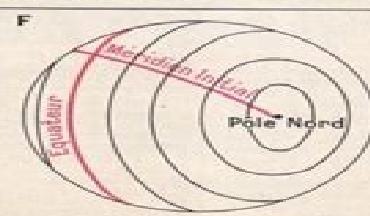
Fig. F. — Autre aspect du globe terrestre, avec le tracé des parallèles, pour un observateur placé face au pôle Nord.
