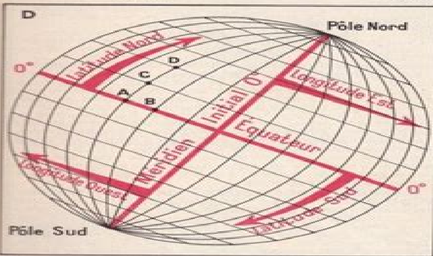
Fig. D. — Le réseau des méridiens et des parallèles se présenterait comme sur cette gravure pour un observateur placé face à l'Équateur. La distance AB est égale à 111 km, 111. La distance CD est égale à 111 km, 111.
