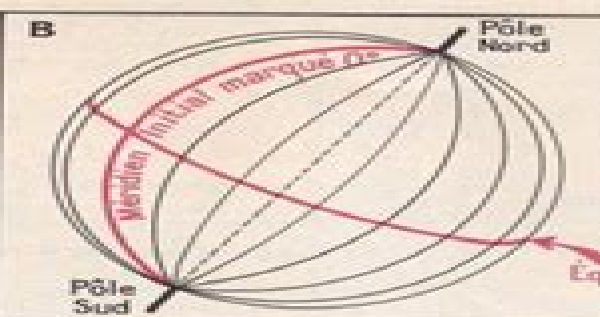
Fig. B. — Elle représente le globe terrestre, tel que le verrait un observateur placé face à l'Équateur, si sur ce globe on avait dessiné le fuseau des méridiens.
