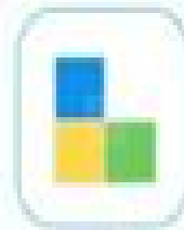
CodeLite
