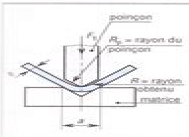
Fig. 2. Pliage en l'air à fond de vè.
