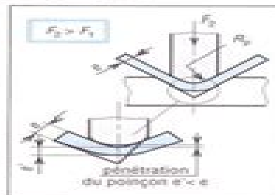
Fig. 3. Pliage (avec frappe).
