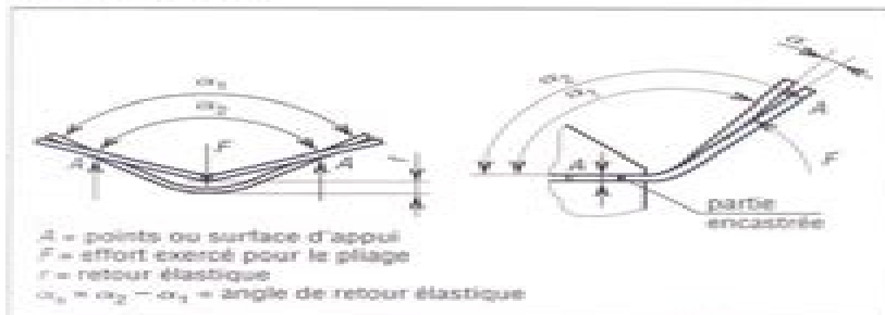
Fig. 1. Exemple de retour élastique de produit plié.
