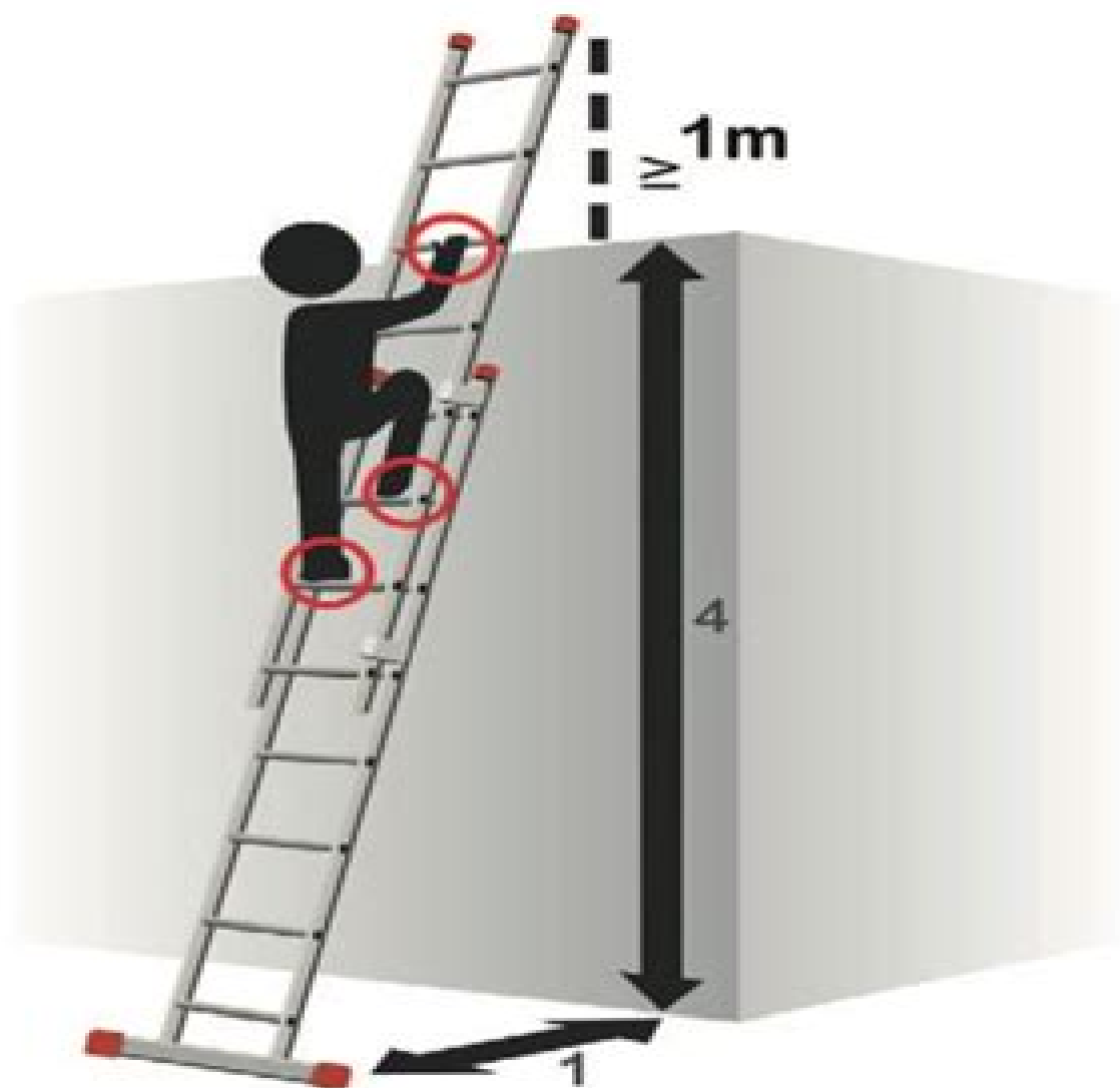
Figura 28. Ejemplo de colocación de una escalera de mano para acceso a un nivel superior.
