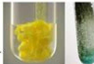
Reacciones de precipitación
