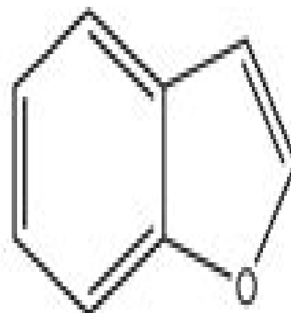
Benzofuran
