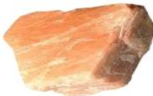
Orthoclase feldspar
