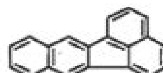
Benzo[k]fluoranthene 252.3 g
