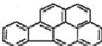
Indeno[1,2,3-c,d]pyrene 276.3 g
