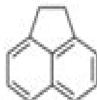
Acenaphthene
