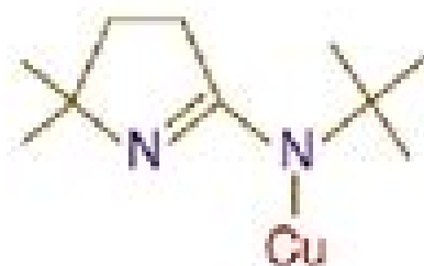
Cu(I)-2-(tert-butylimino)-5,5'-dimethylpyrrolidinate (2)
