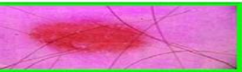
Benign
