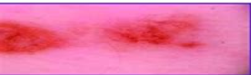
Benign
