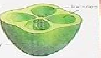
ovule
