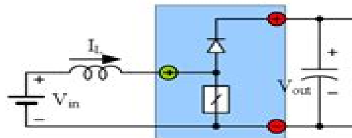
(d) N-cell boost converter
