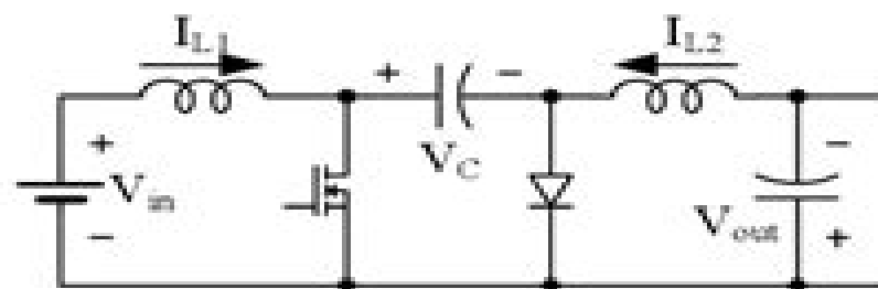
(g) Cuk converter
