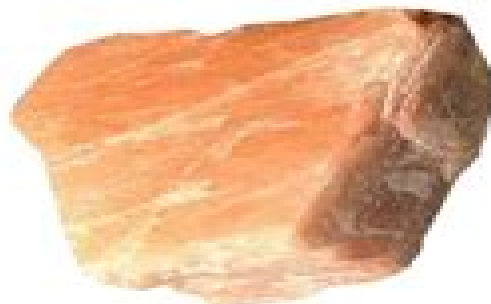
Orthoclase feldspar
