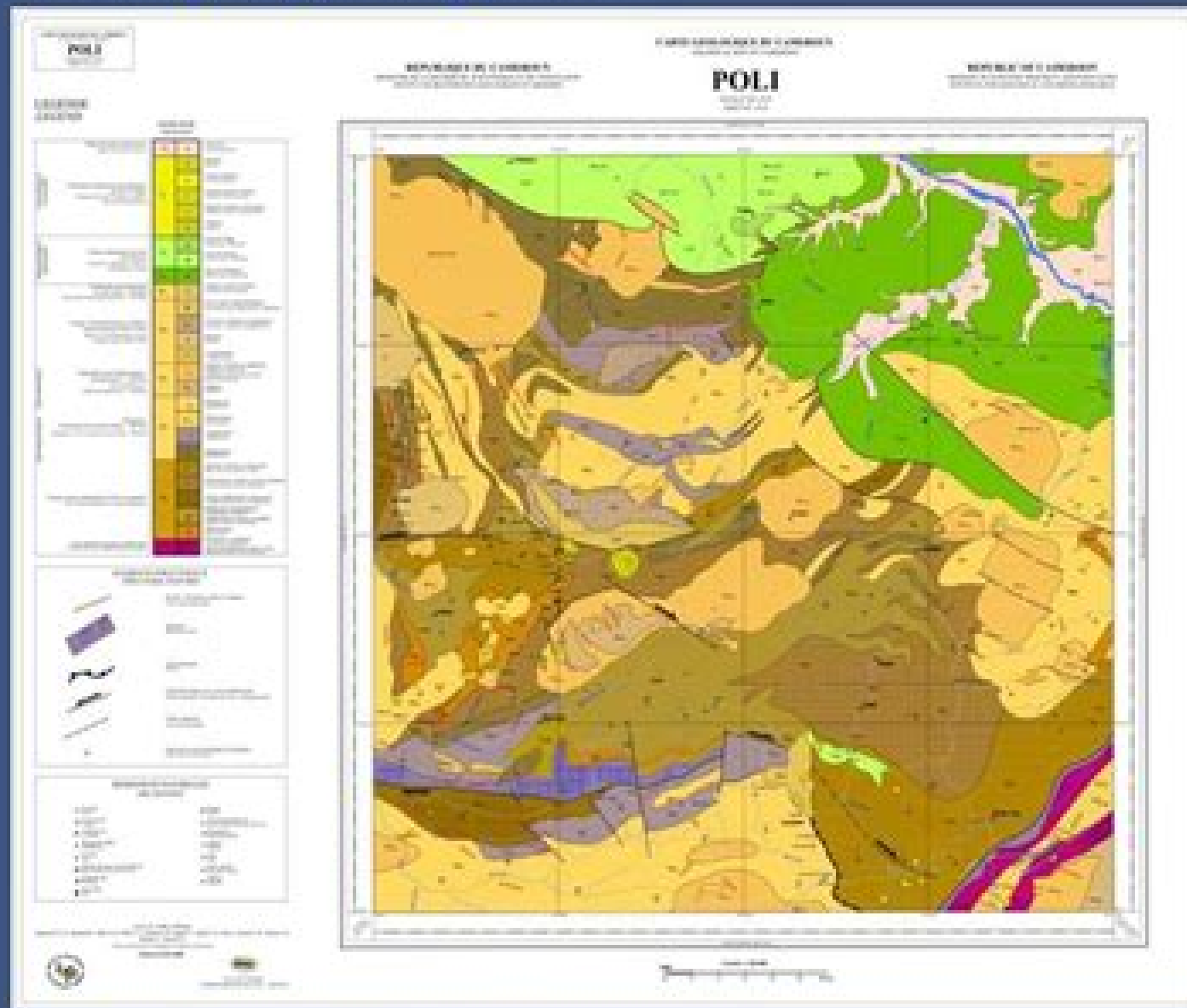
Carte géologique du Cameroun à 1/200000: feuille de Poli
