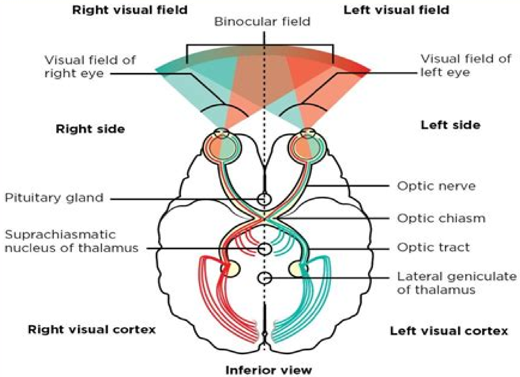
Fig 5. Visual pathways
