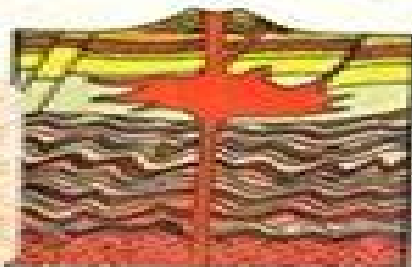
garnet
