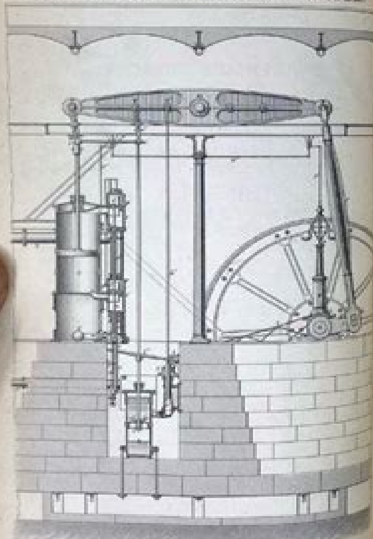
Longitudinal Section
