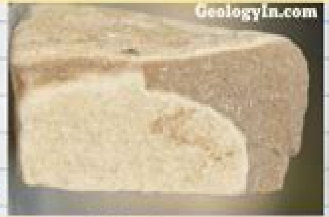
Mudstone
