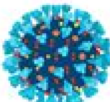
SARS 120nm
