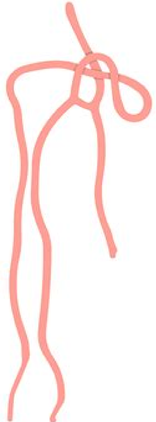
Ebola virus 80x970nm
