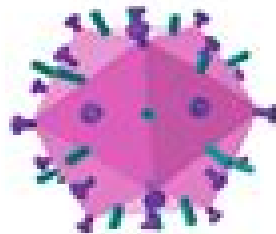
HIV-1 120nm
