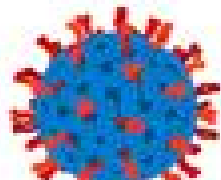
Rotavirus 80nm
