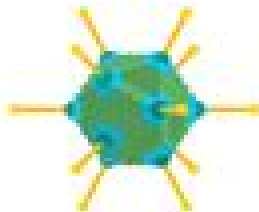
Adenovirus 90nm
