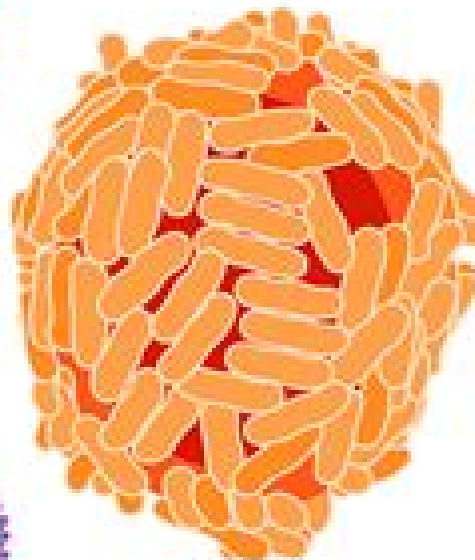
Variola virus 360nm
