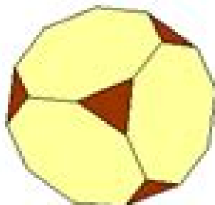
abgestumpftes Hexaeder
