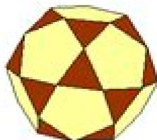
Ikosidodekaeder
