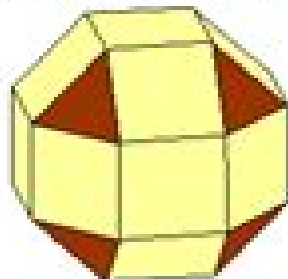
Rhombenkuboktaeder
