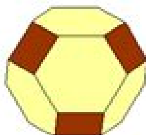
abgestumpftes Oktaeder
