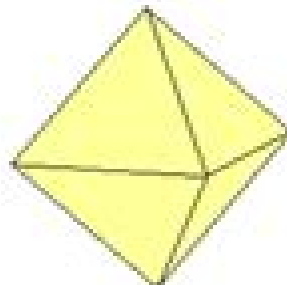
Oktaeder
