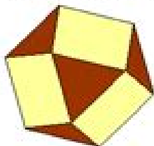
Kuboktaeder
