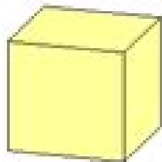
Würfel (Hexaeder)
