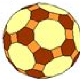
abgestumpftes Ikosidodekaeder
