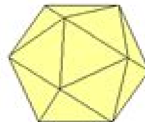
Ikosaeder
