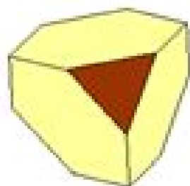
abgestumpftes Tetraeder
