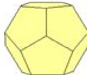
Dodekaeder
