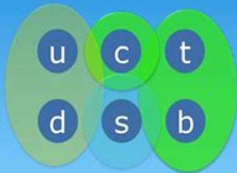
quarks
