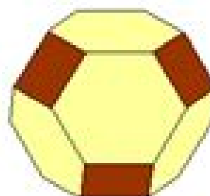
abgestumpftes Oktaeder
