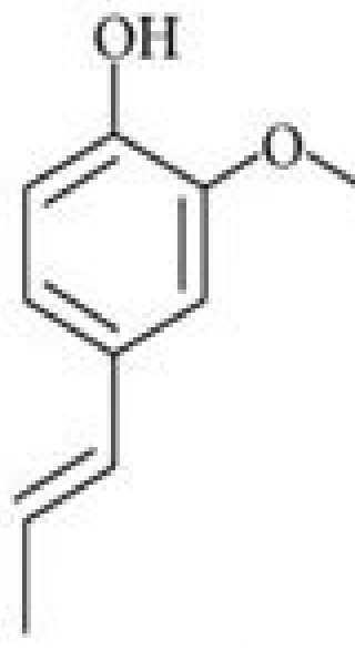
Isoeugenol
