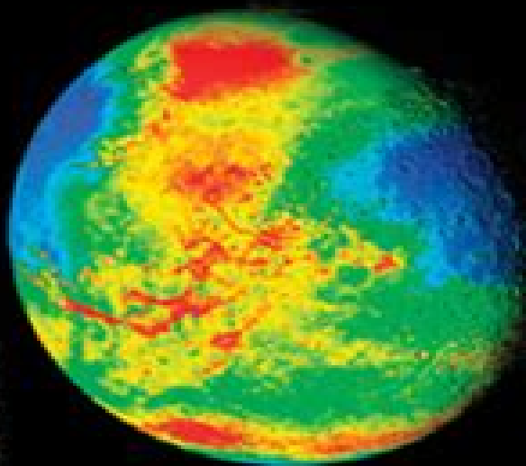
Thermal Inertia
