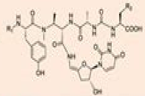
Pacidamycin
