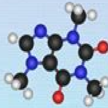
Caffeine
