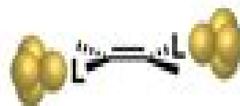
Alkene
