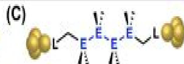
Oligometallane
