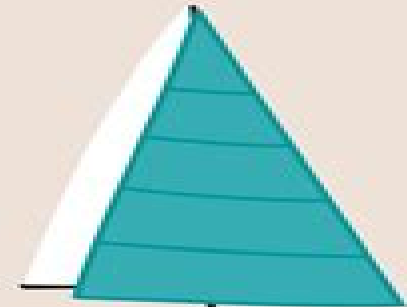
GENOA
