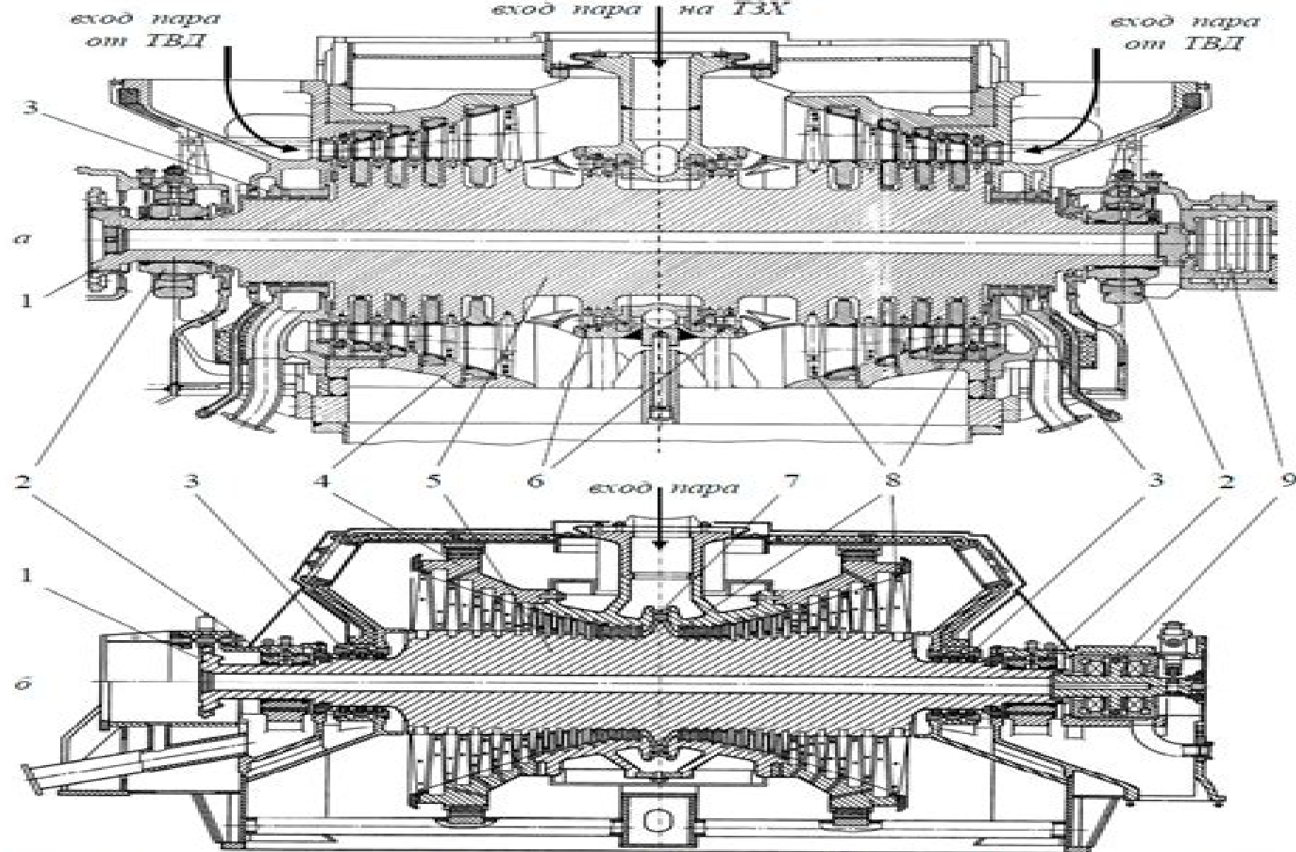
Рис. 53. Активная паровая турбина (турбина низкого давления ТВ-12) со сходящимися потоками пара (а) и реактивная однокорпусная турбина атомного ледокола с расходящимися потоками пара и центробежной регулировочной ступенью (б).
