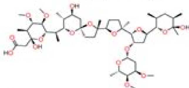
Maduramycin C_{47}H_{80}O_{17} MW 917.13
