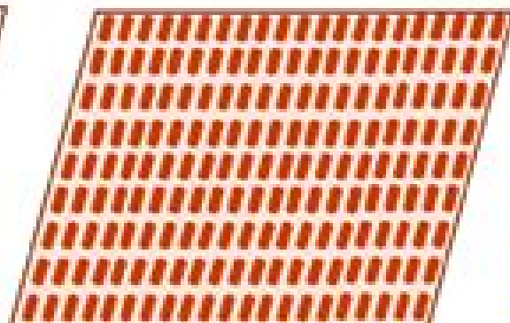
Crystalline
