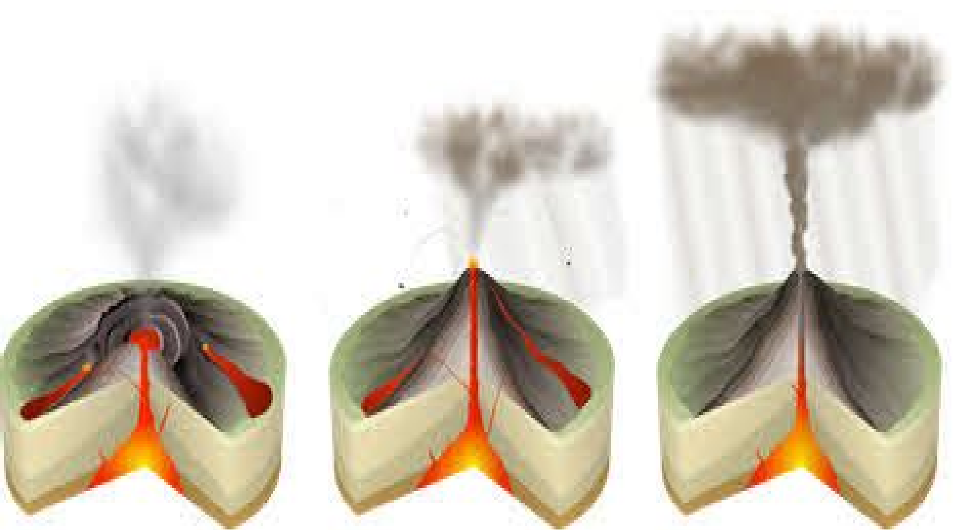
Эффузивное
