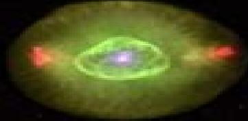
Little Ghost Nebula (NGC 6389)
